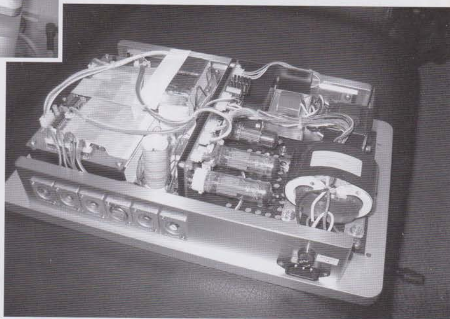
△ Zanden 5000 最特別之處是使用飛利浦TDA1541A雙「皇冠」DAC及不用數碼式濾波器。
